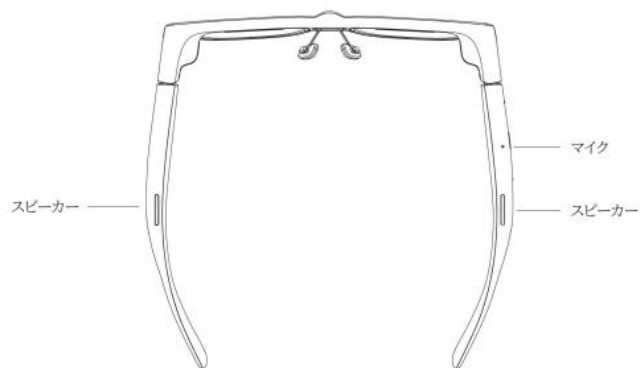
上面
